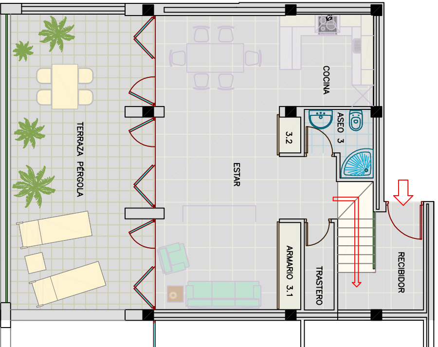
PLANTA INFERIOR
