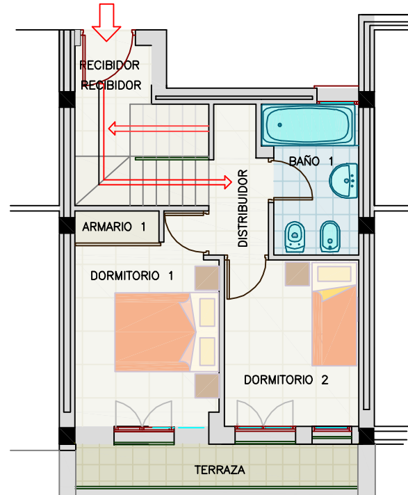
PLANTA SUPERIOR
