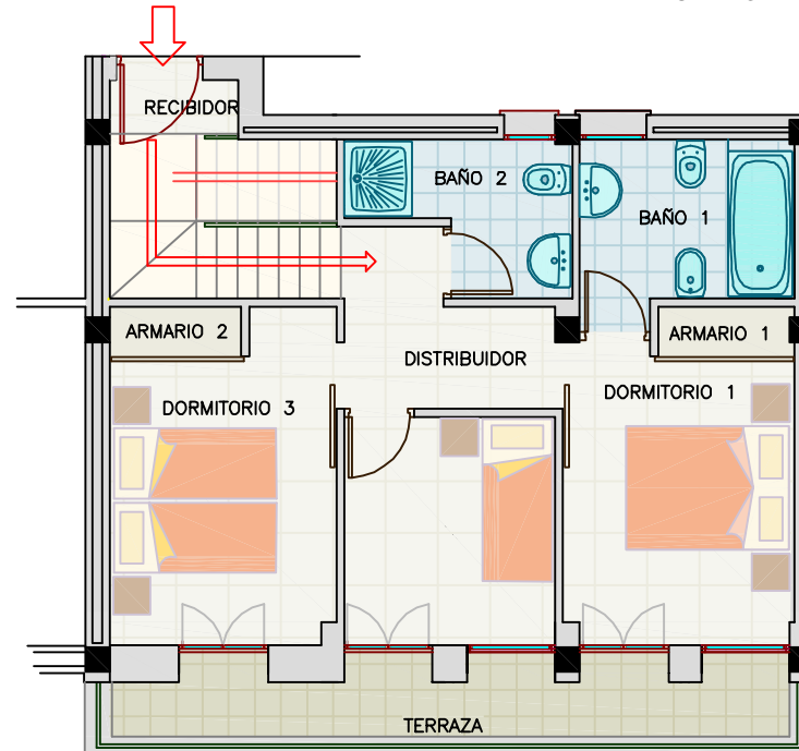
PLANTA SUPERIOR
