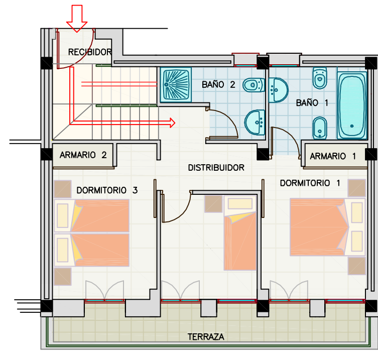
PLANTA SUPERIOR
