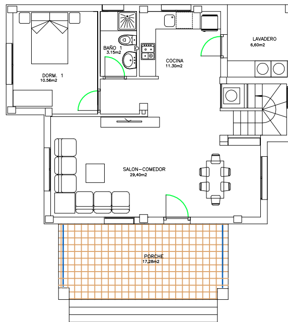
PLANTA BAJA
