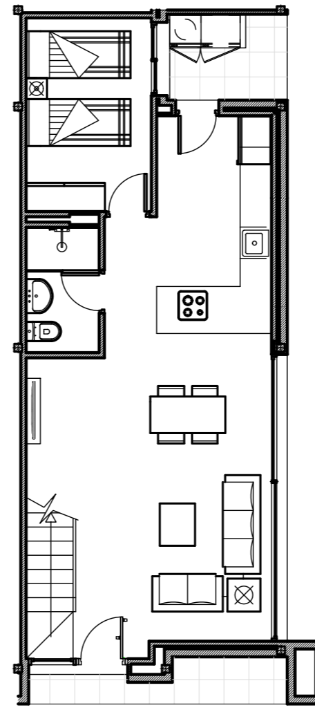
PLANTA BAJA
