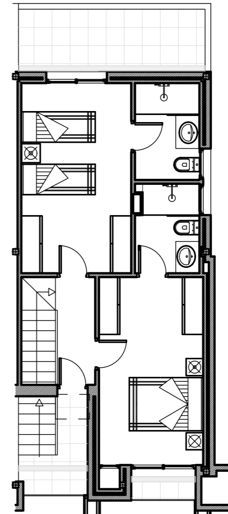
PLANTA ALTA
