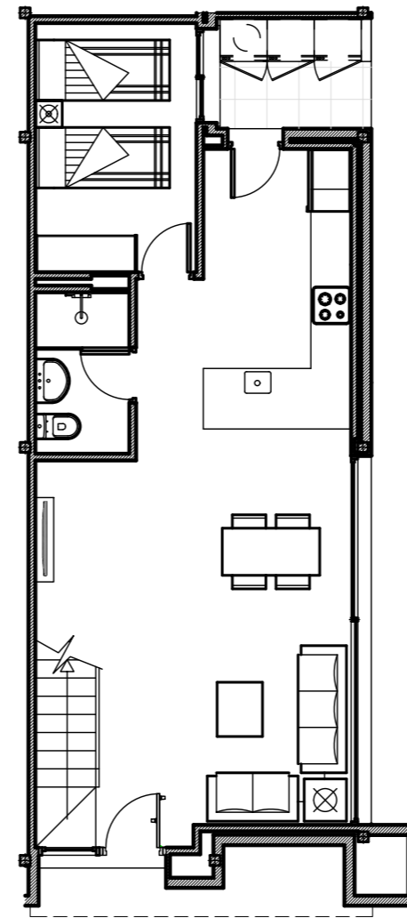
PLANTA BAJA
