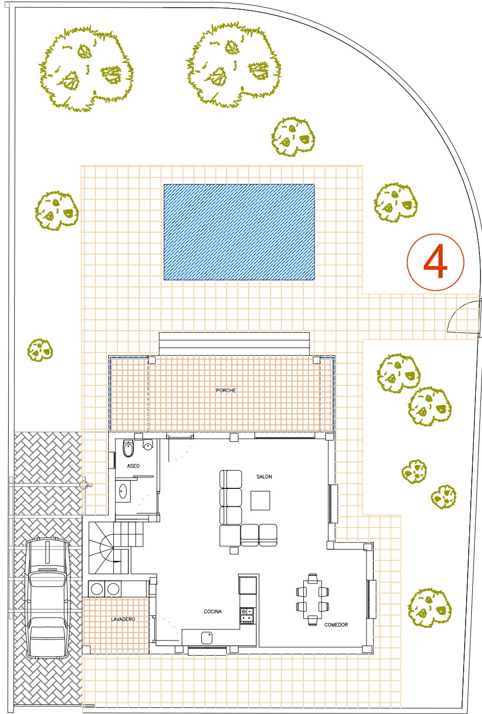
CONJUNTO PARCELA 4 PLANTA BAJA
